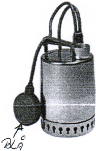
Grundfos kælderpumpe KP150A-1 m/svømmeafbryder
